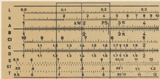
Fig. 32 Omrekening: 19.5 \text{ kW} \approx 26.5 \text{ PK} N. B. Op de liniaal wordt PK (paardekracht) aangeduid met PS (Pferdestärke)
