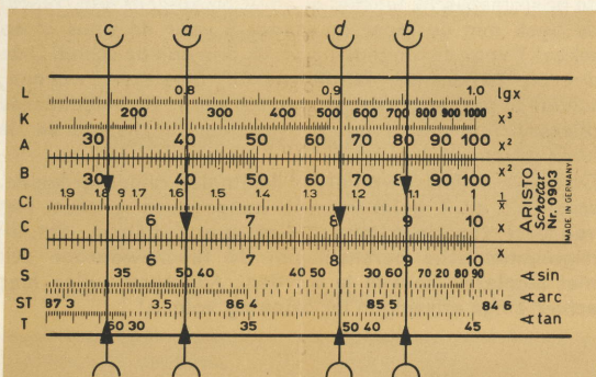
Fig. 19 a) \tan 32.4^\circ = 0.635 aflezen op D b) \tan 48^\circ = 1.111 aflezen op CI met de schuif in de oorspronkelijke stand c) \cot 29.3^\circ = 1.782 aflezen op CI met de schuif in de oorspronkelijke stand d) \cot 51^\circ = 0.810 aflezen op D
