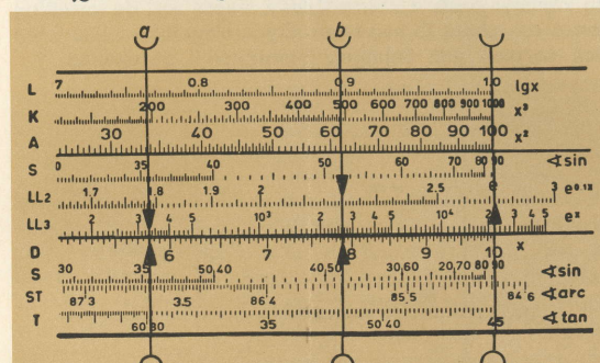
Fig. 28 Natuurlijke logarithmen (grondtal e) a) \ln 330 = 5.80 b) \ln 2.2 = 0.788
