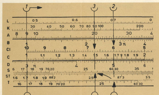
Fig. 22 De rechthoekszijden (katheten) zijn bekend
